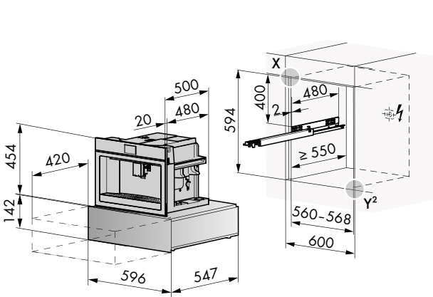
Sopra coffee center h 454 Sotto scaldavivande o sottovuoto h 142
