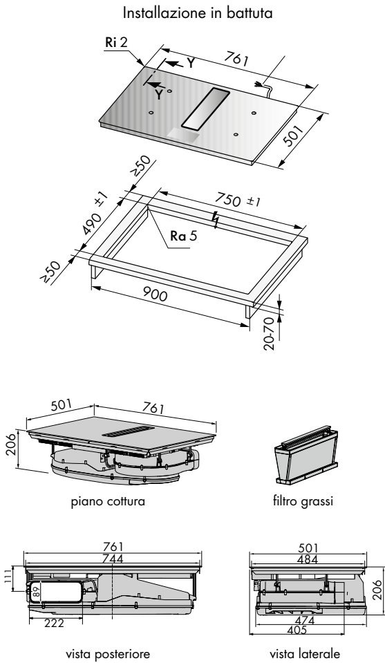
Dimensioni prodotti/vano incasso
