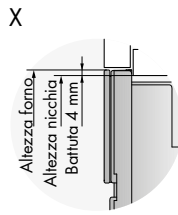
Dettaglio dimensioni Coffee-Center
