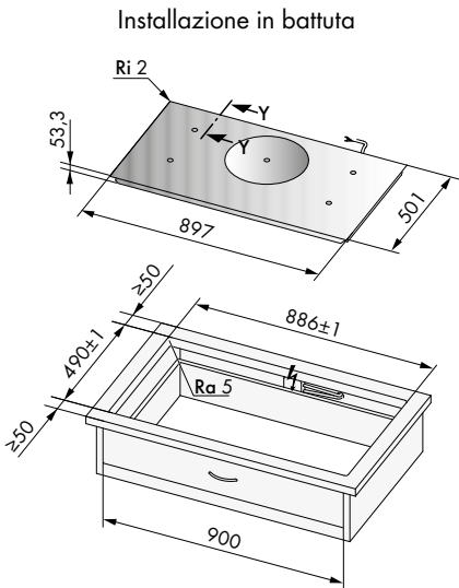
Dimensioni prodotti/vano incasso
