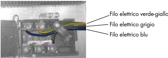
Schema allacciamento elettrico monofase (morsettiera)
