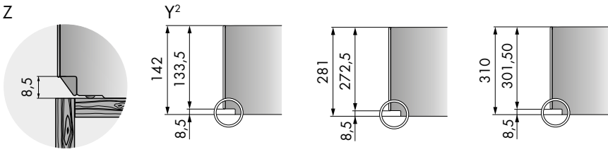
Dettaglio dimensioni cassetti
