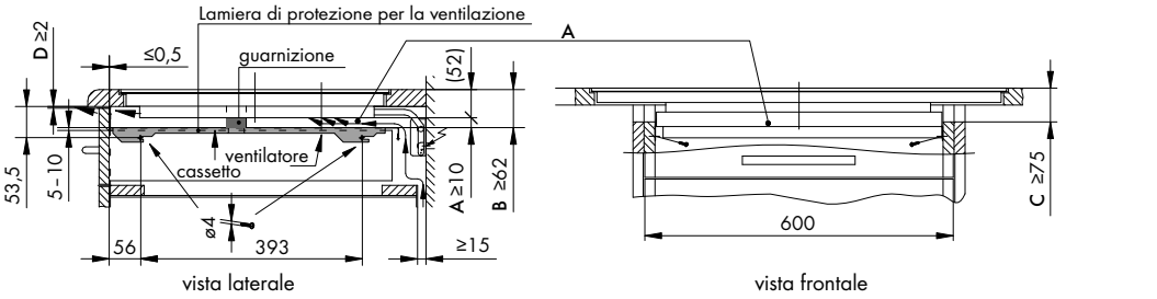
Piano cottura: MAXIFLEX V6000 I905 CTI6T95MMSOLD (lamiera H61085)
