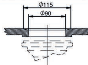
FORO SCARICO LAVELLO/ SINK DRAIN HOLE
