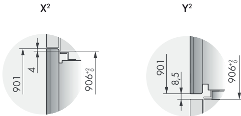
Dettaglio dimensioni
