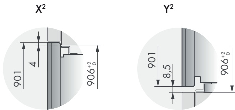
Dettaglio dimensioni
