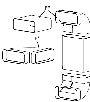
F. Canali piatti, varianti di curve e raccordi (versione aspirante)
