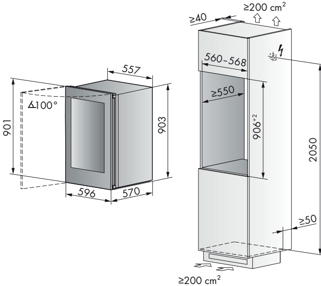
Dimensioni prodotti/vano incasso
